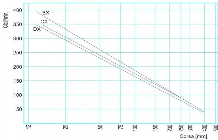
Diagramma cicli/minuto
